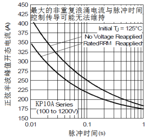
Fig. 6 - 最大反向浪涌电流
