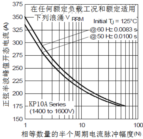
Fig. 12 - 最大反向浪涌电流
