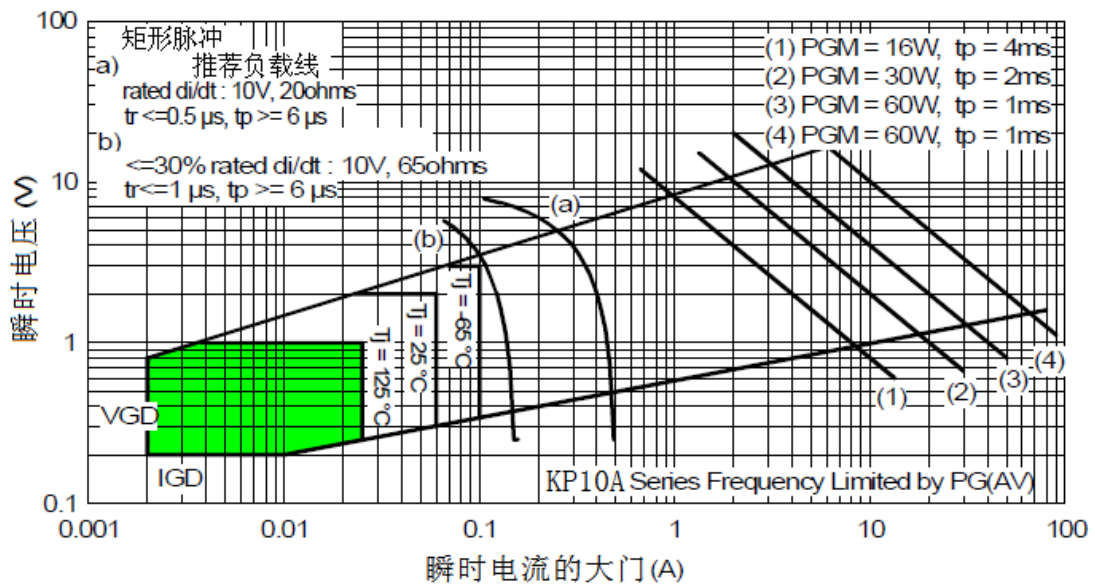
Fig. 16 - 栅极特性
